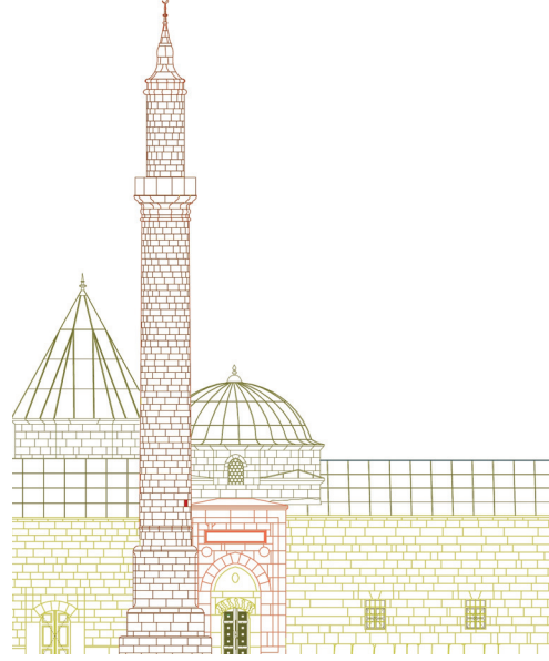
Ahi Evran Zaviyesi (cephe çizimi)
